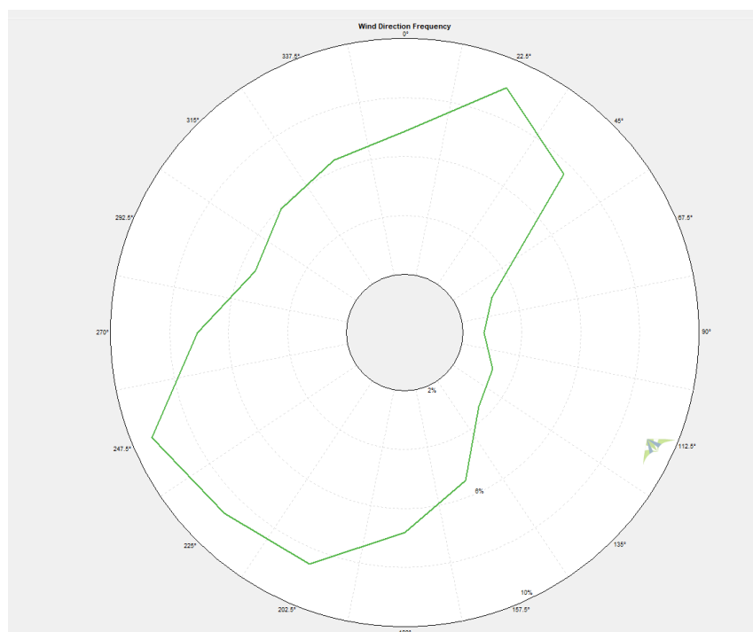
Figure 5 : Rose des vents (source : NORDEX, 2019)
